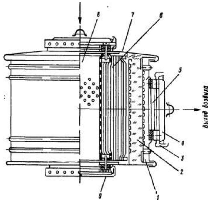
1 — корпус; 2 — шихта, 3 — кольцо ниппельное; 4 — заглушка с ручкой; 5 — боковое отверстие; 6 — фильтр противодымный, 7 — крышка верхняя; 8 — каркас фильтра, 9 — доньшко
