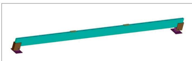
Рис. 1. Модель стеклянной балки
